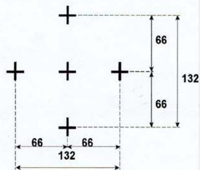
Das Kegelbild
